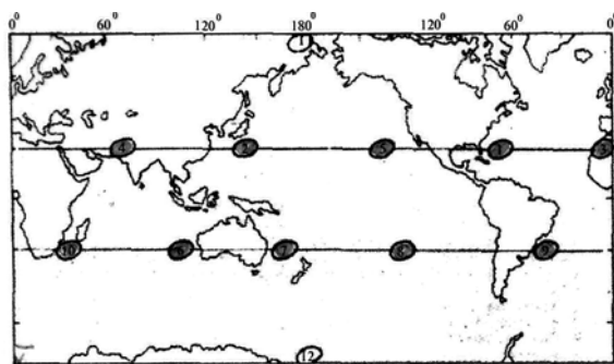
Рис. 1. Пояс дьявола на 30-х параллелях северной и южной широт (по А. Сандерсону).
