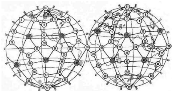
Рис. 2. Икосаэдро-додекаэдрический силовой каркас Земли («русская сетка»).
